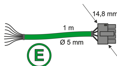
WH3-INP-100-G08-TAP-01 wiązka sygnałów wejściowych
