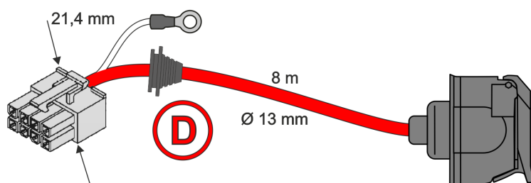
WH3-OUT-800-G08-PVC-01-STD wiązka gniazda haka
