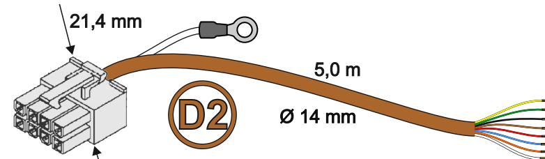
WH3-OUT-G08-500-G08-P13-01 wiązka przedniego gniazda haka
