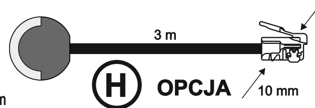
LED-RGY-300-R09-CLR-01 3-kolorowa dioda sygnalizacyjna
