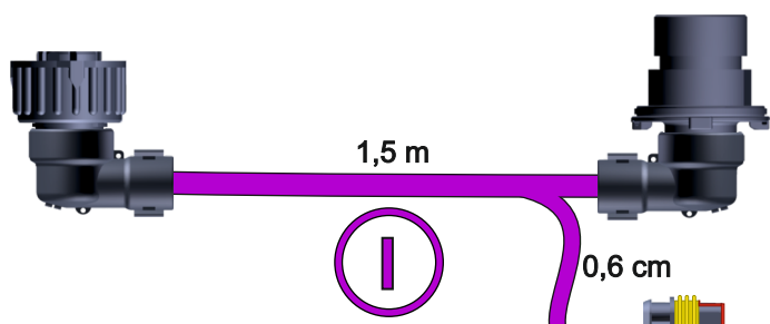
LMP-EXT-150-P2P-P10-LFT-02-STD przedłużacz lewej lampy z wyprowadzonymi sygnałami P2P
