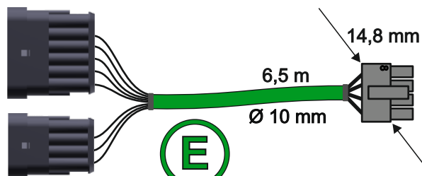
WH3-INP-G08-650-P2P-P10-01 wiązka sygnałów wejściowych P2P
