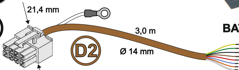
WH3-OUT-300-G08-P14-01 wiązka przedniego gniazda haka
