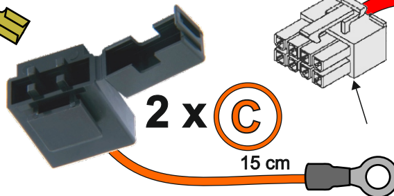
BAT-FSE-015-G08-CLR-01 wiązka bezpiecznika
