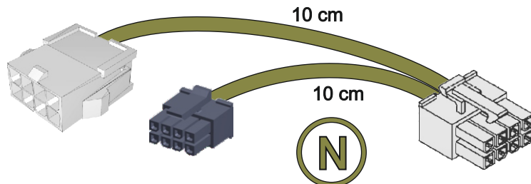
WH3B-SPR-020-1T2-CLR-01 Wewnętrzny rozgałęziacz sygnału wyjściowego
