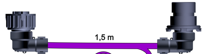
WH3-INP-650-P2P-P10-01 wiązka sygnałów wejściowych P2P
