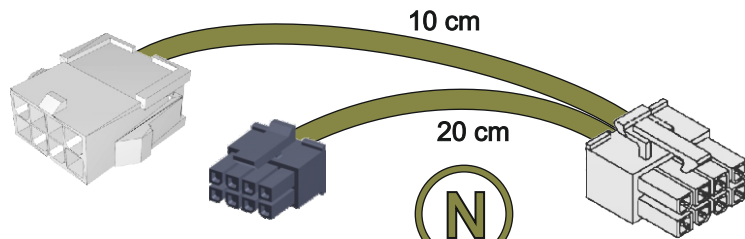
WH3B-SPR-020-1T2-CLR-01 Rozgałęziacz sygnału wyjściowego modułu WH3Q-DS
