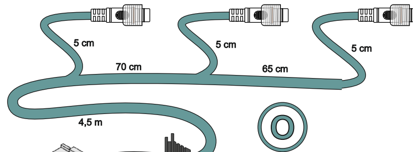
LMP-BLK-450-70-60 Wiązka zasilania lamp na belce i świateł obrysowych
