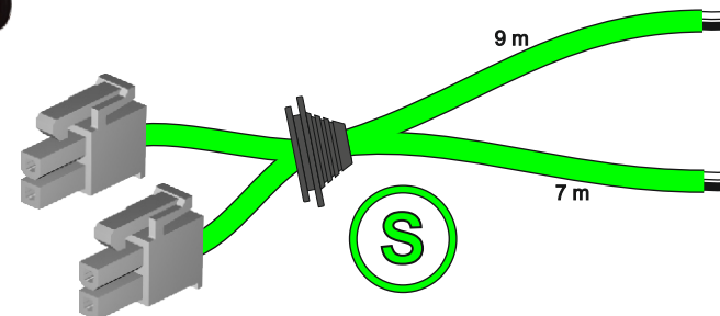
LMP-OBR-700-900 Wiązka zasilania świateł obrysowych OPCJA
