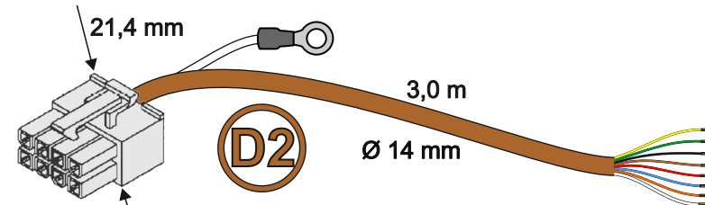
WH3-OUT-G08-300-G08-P13-01 wiązka przedniego gniazda haka
